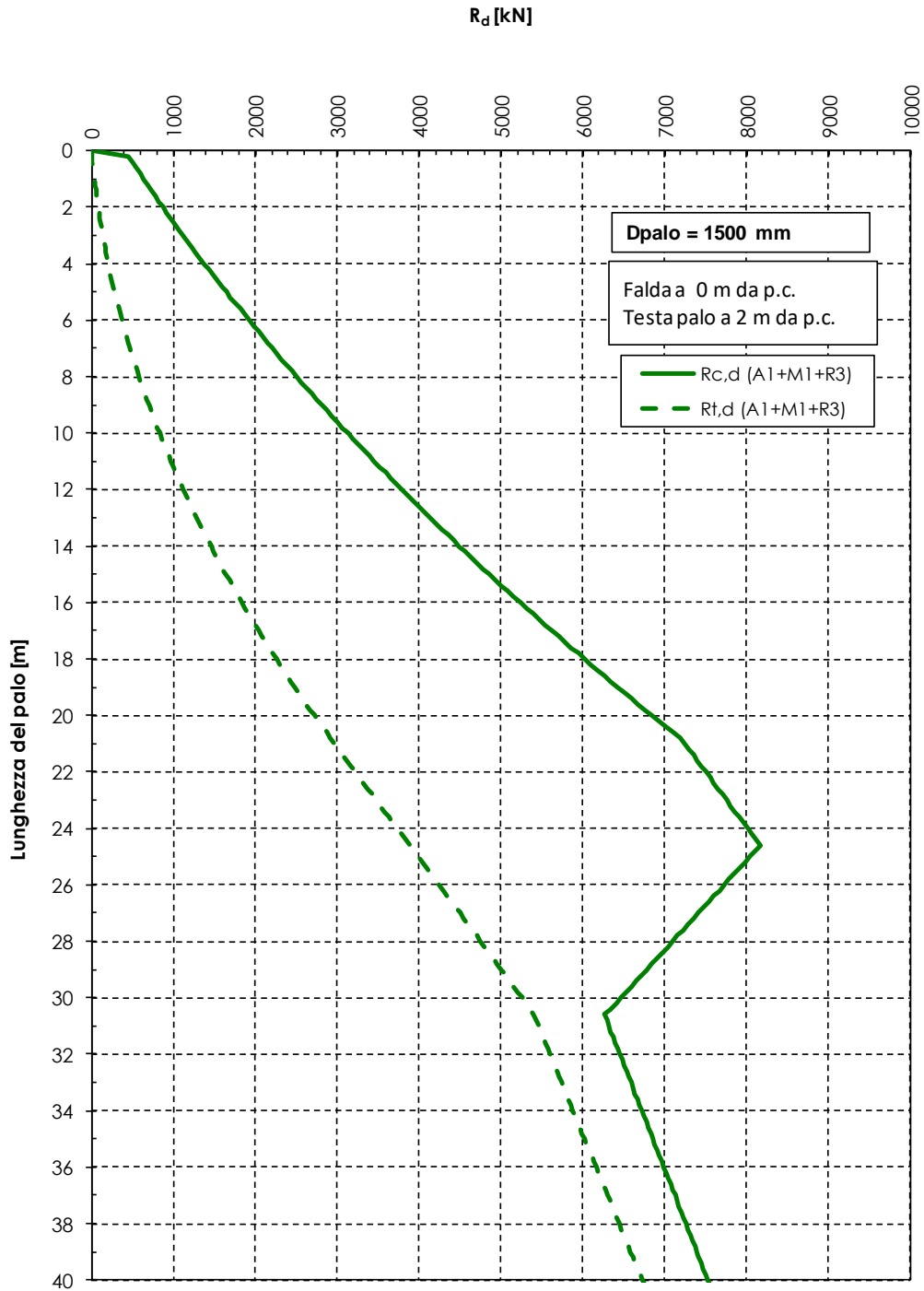
Ponte ferroviario su Canale Ozzoretto - km 41+195
