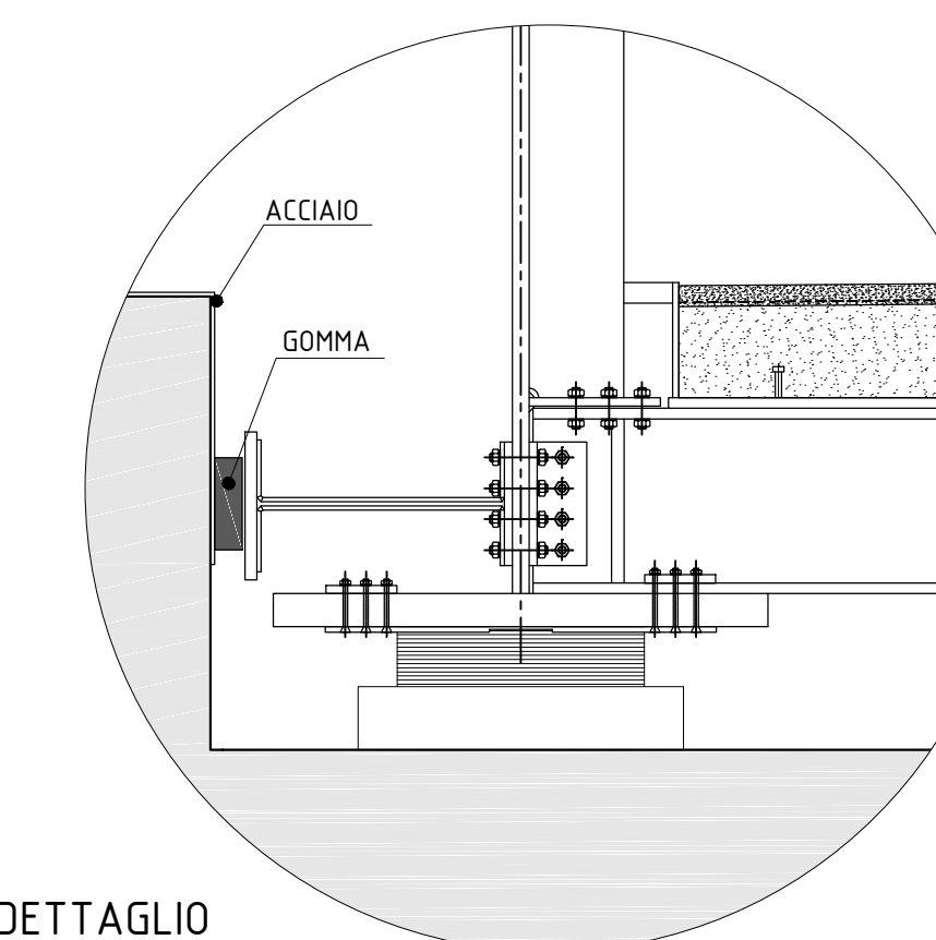
DETTAGLIO RITEGNO SISMICO SCALA 1:20
